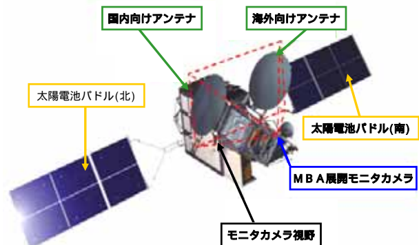
「きずな」MBA展開モニタ用カメラ位置((C)JAXA)
